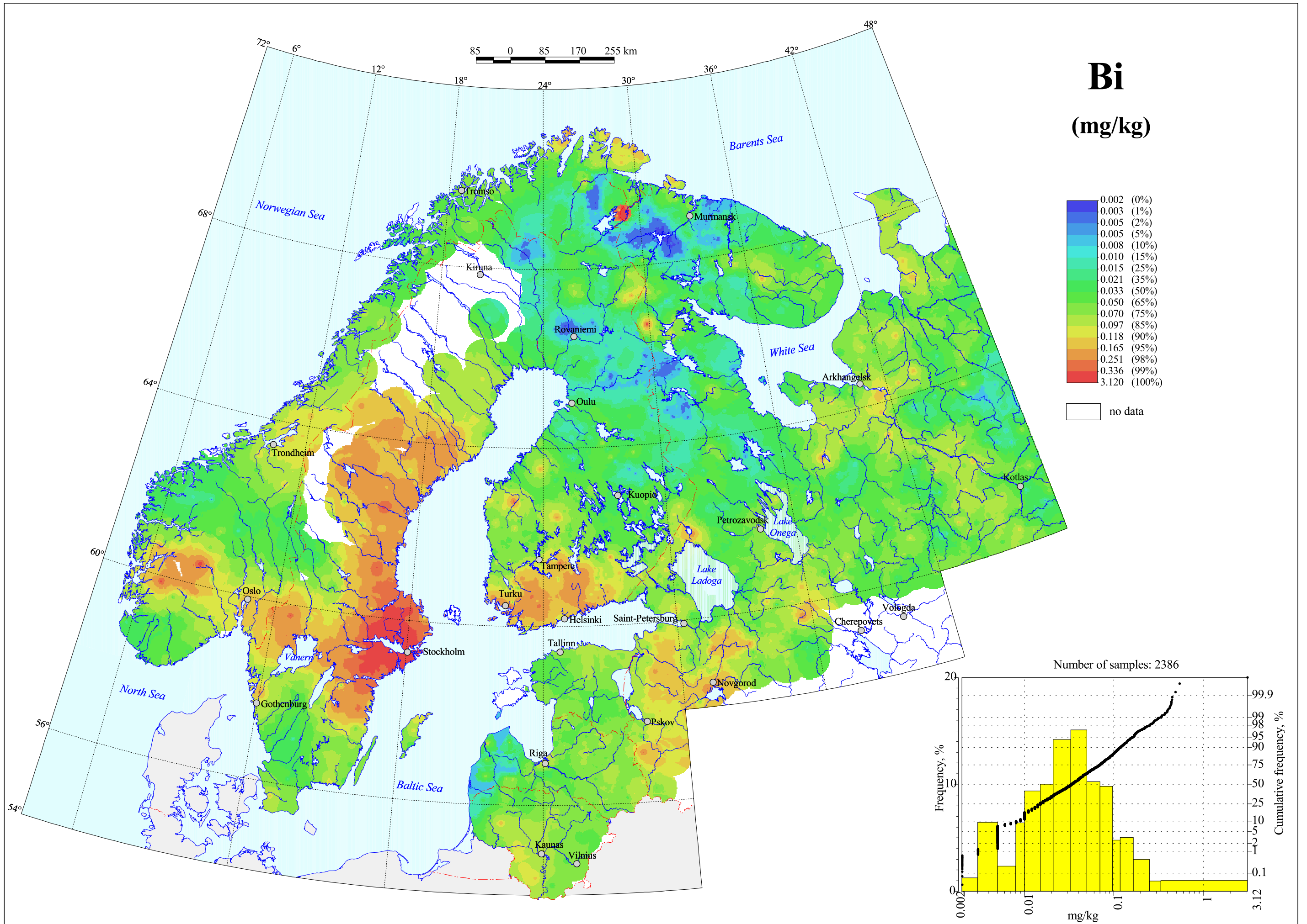
Bismuth in C-horizon, Grain Size <2 mm, Aqua regia Extraction
